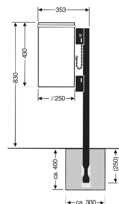
Modello 20 O per installazione fissa con tubo d'acciaio
