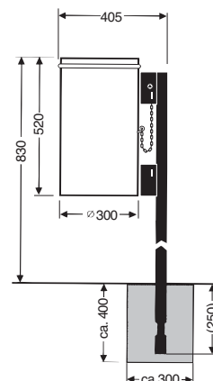
Modello 35 O per installazione fissa con tubo d'acciaio
