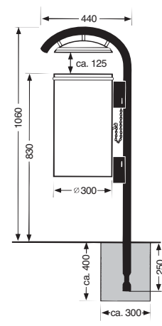
Modello 35 O-D per installazione fissa con tubo d'acciaio
