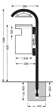
Modello 20 O-A-D per installazione fissa con tubo d'acciaio
