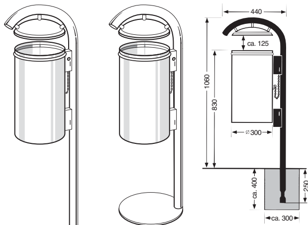
Modello 35 O-D per installazione fissa con coperchio
