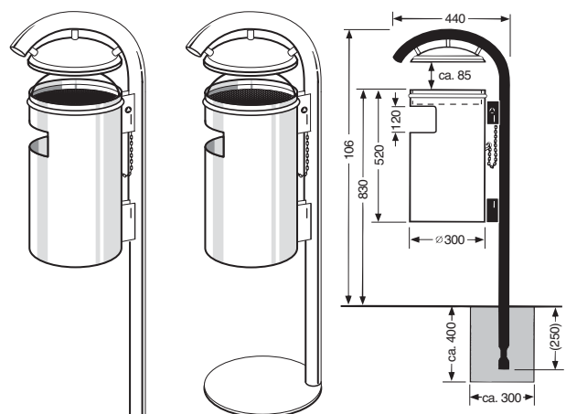
Modello 35 O-A-D per installazione fissa con tubo d'acciaio
