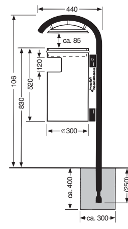
Modello 35 O-A-D per installazione fissa con tubo d'acciaio
