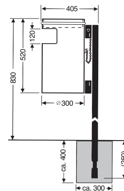
Modello 35 O-A per installazione fissa con coperchio
