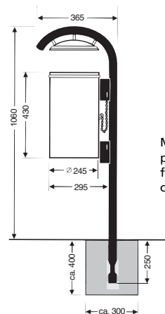
Modello 20 O-D per installazione fissa con tubo d'acciaio
