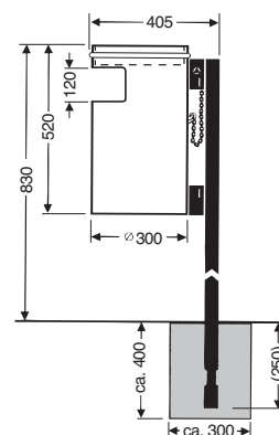
Modello 35 O-A per installazione fissa con tubo d'acciaio
